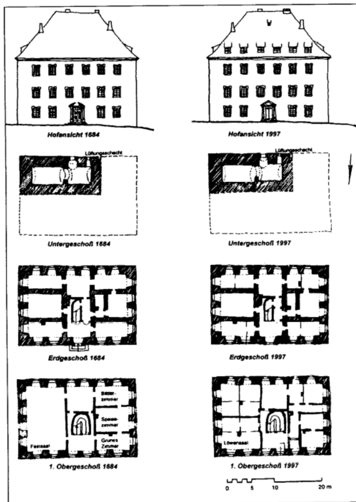
Hirschberg: Auf- und Grundriss des Schlosses Hirschberg im Zustand von 1684 und 1997 (Löffler 2000, Abb. 170).
